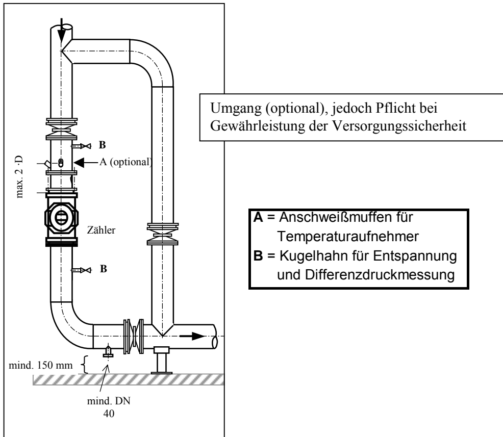
Bild 4: Installationsvorschrift für DKZ
