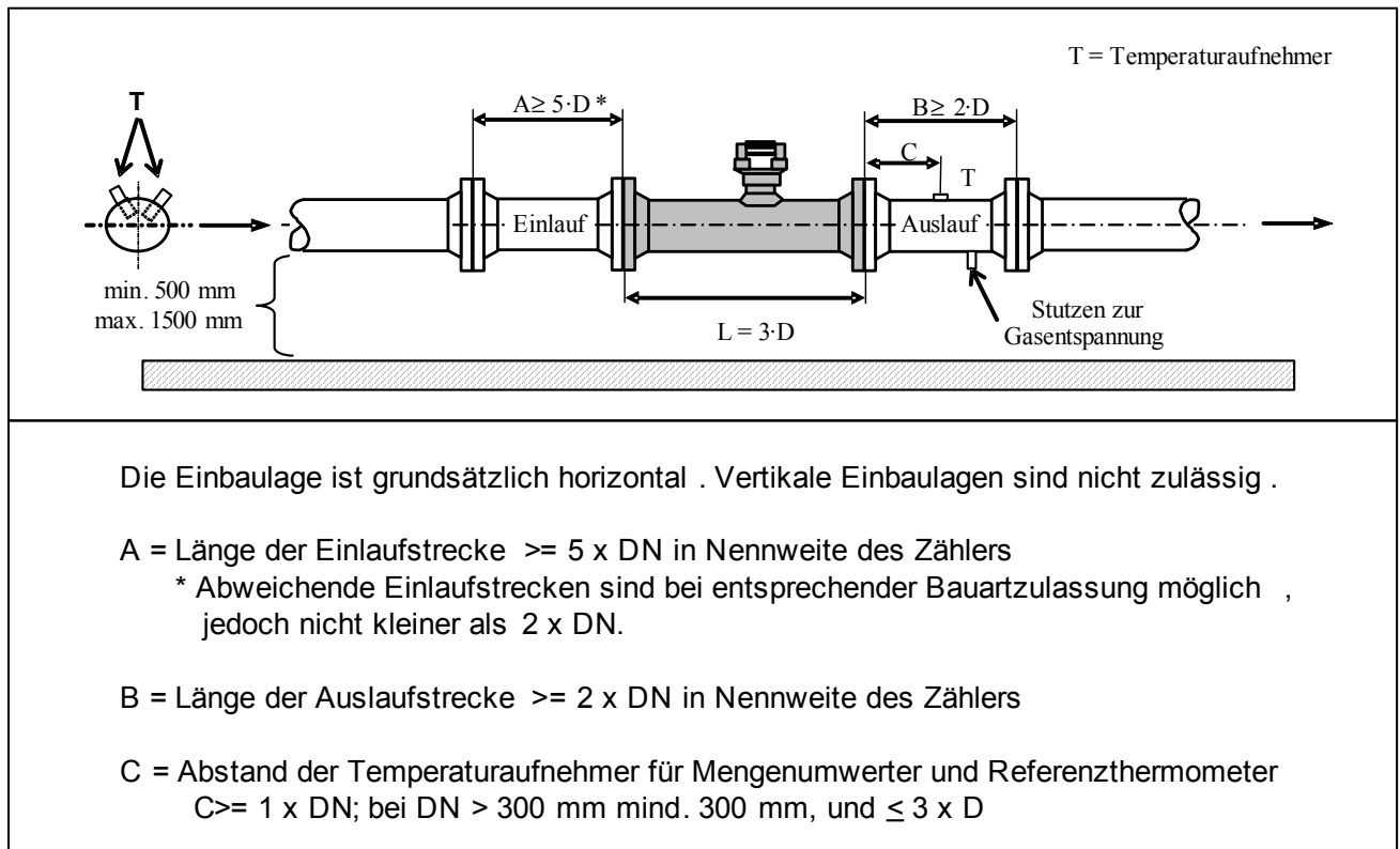
Bild 5: Installationsvorschrift für TRZ
