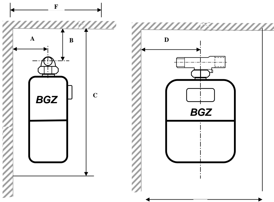
Bild 1: Maße BGZ
