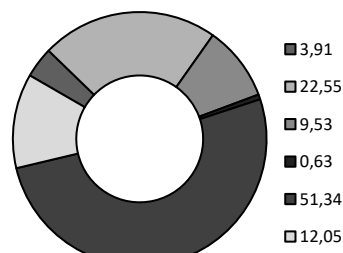
Verbleibender Energieträgermix
