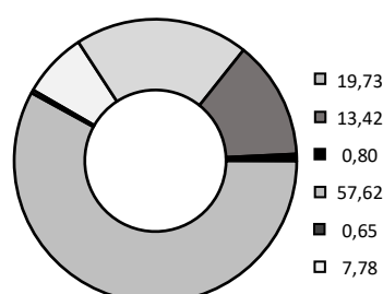
Verbleibender Energieträgermix
