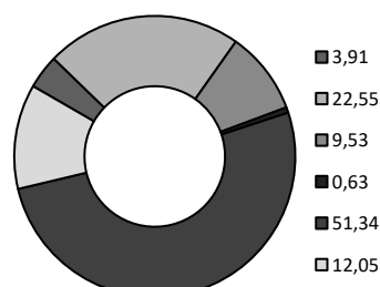
Verbleibender Energieträgermix
